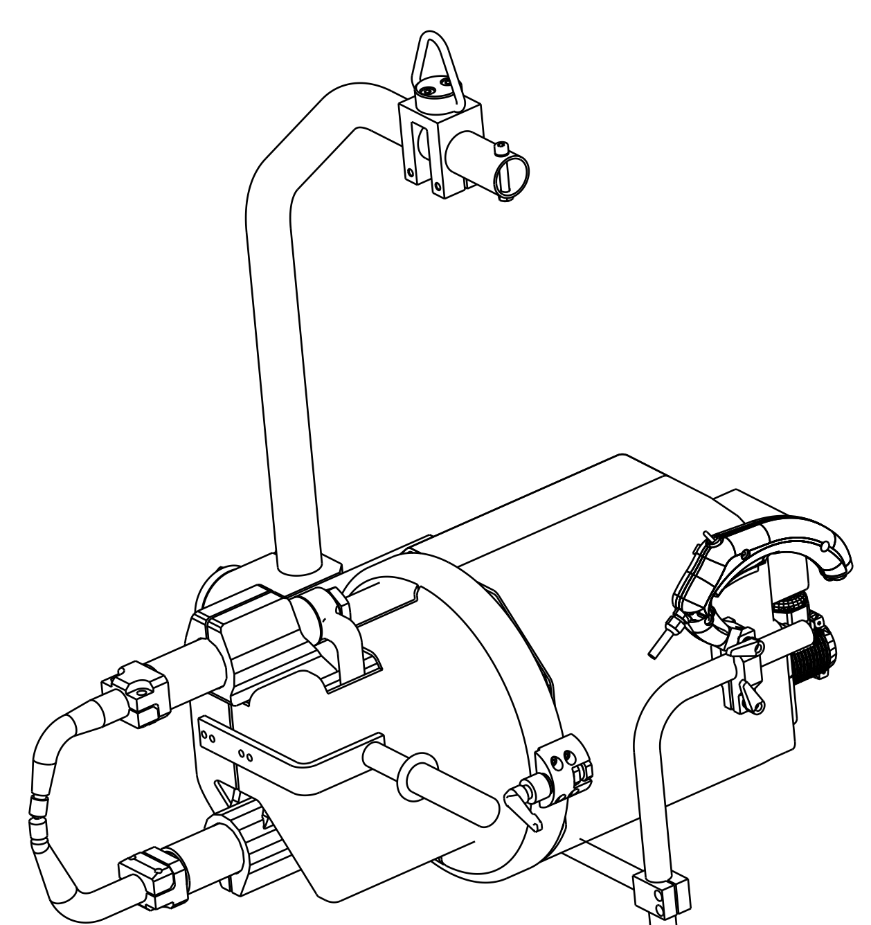
Isometric view Scale: 1:5
